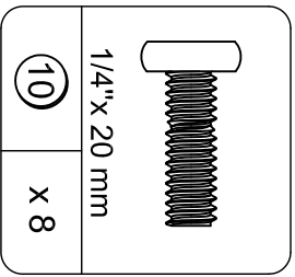
BOLT TCS1114
